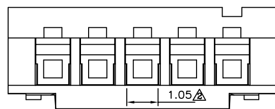
△ 02~05 Pin
