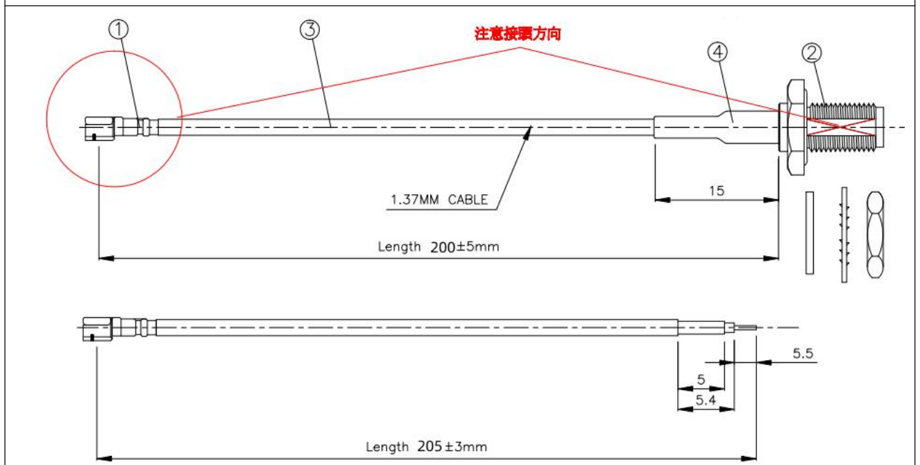
产品结构图
