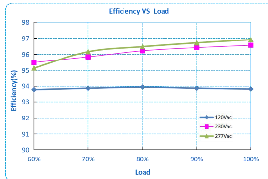
R3-320Y ( I_o=1.2A )
