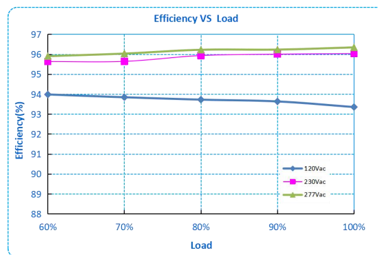
R3-240Y ( I_0=1.0A )
