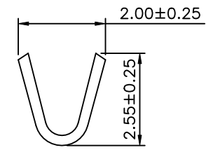
△ A-A Section
