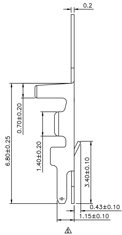
△ A-A Section
