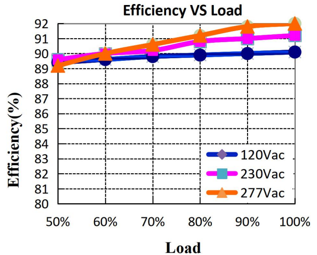
MTP-120X068-OF(Io=1.77A)
