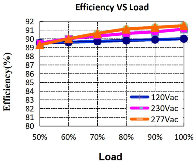
MTP-120X068-OF(Io=2.15A)
