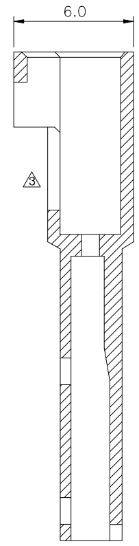
Section A-A
