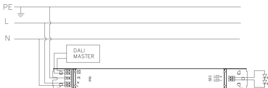
Fig. A: DALI Dimming
