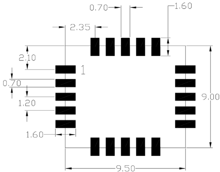
Fig. 2.2 PCB pad
