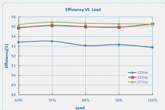
F2-240D-343 ( I_o=1.05A )
