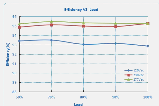
F2-240D-228 ( I_o=1.05A )
