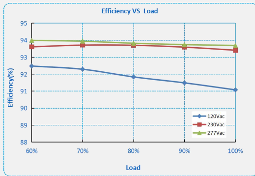
F2-240D-054 ( I_o=6.67A )
