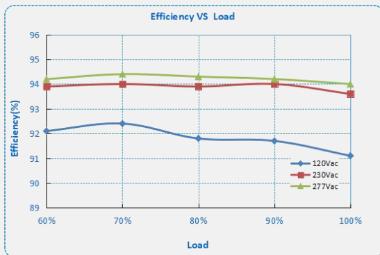
F2-240D-228 ( I_o=1.5A )
