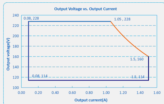
F2-240D-228
