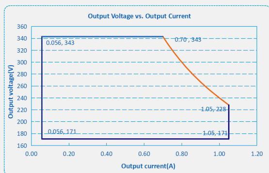
F2-240D-343
