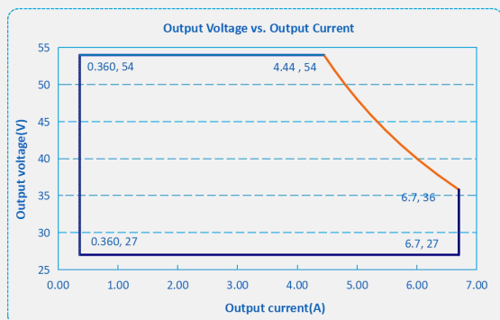
F2-240D-054
