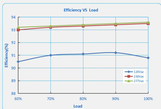
F2-200X-143 ( I_o=2.2A )
