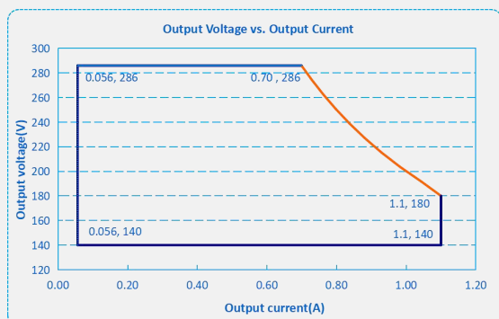
F2-200D-286
