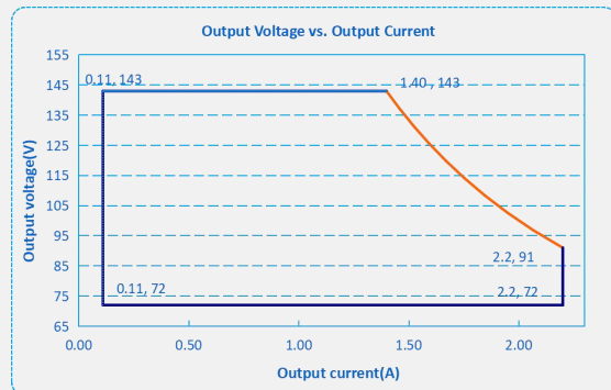
F2-200D-143
