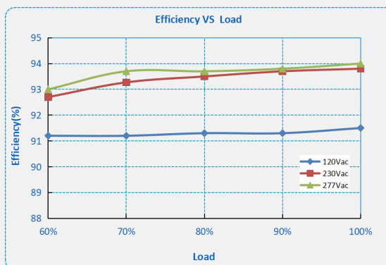
F2-200X-143 ( I_o=1.4A )
