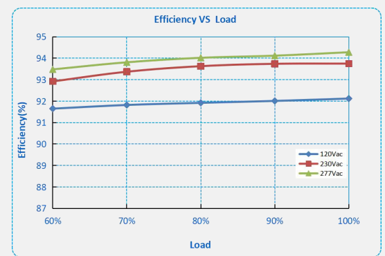
F2-200X-286 ( I_o=1.1A )
