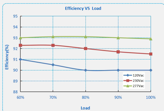
F2-200X-054 ( I_o=5.55A )
