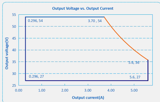
F2-200D-054
