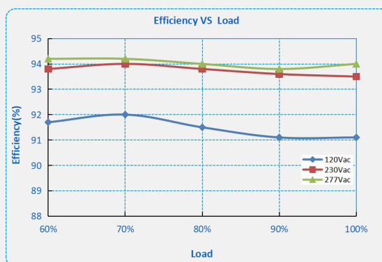
F2-200X-054 ( I_o=3.7A )
