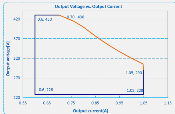
F1E-320X-430
