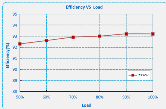
F1E-320X-056 ( I_o=5.7A )
