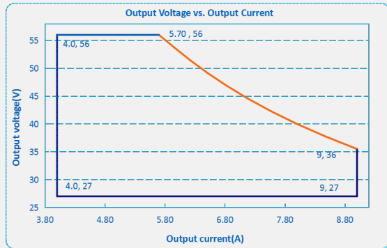
F1E-320X-056
