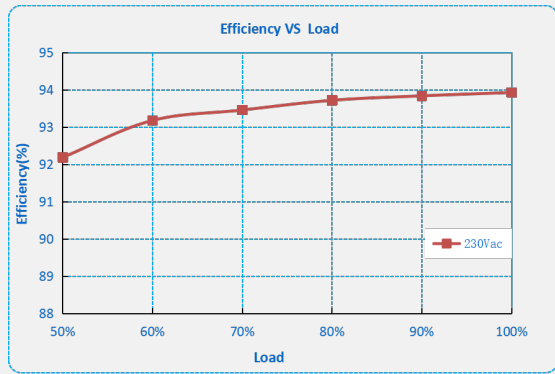
F1E-150X-214R ( I_o=0.70A )
