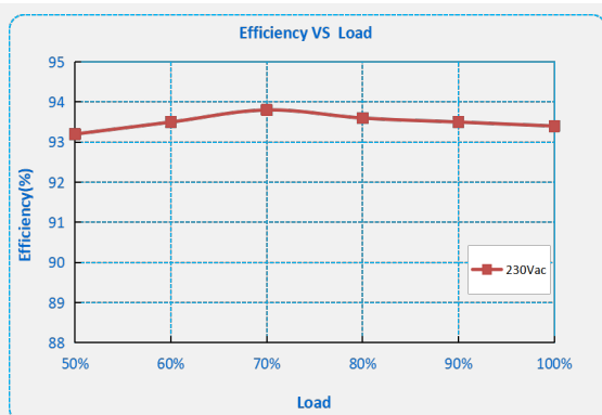
F1E-150X-054R ( I_o=2.95A )
