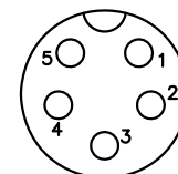
5 PIN(ø2.0 7A)
