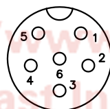
6 PIN(ø1.2 5A)
