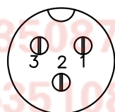
3 PIN(ø2.5 7A)
