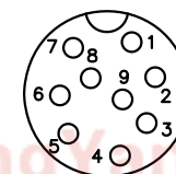
9 PIN(ø1.2 5A)
