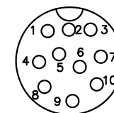
10 PIN(ø1.2 5A)
