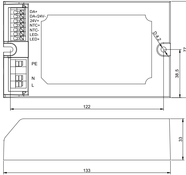
DL-80H-V115GX-MXK
