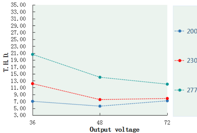
T.H.D. VS Output voltage(DL-50H-V72P-MXC)
