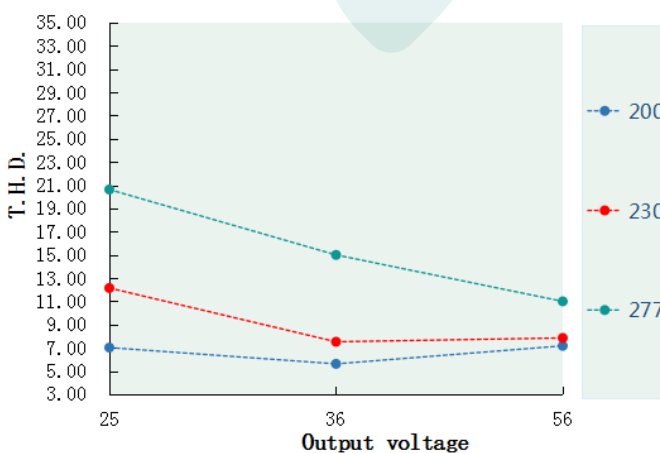
T.H.D. VS Output voltage(DL-50H-V56P-MXC)
