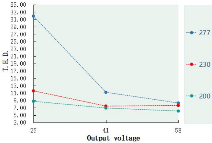
T. H. D. VS Output voltage(DL-40H-V58GX-MXK)
