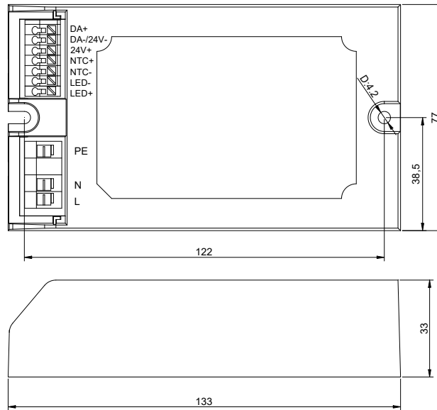
DL-110H-V158GX-MXK
