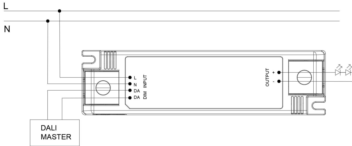
Fig. A: DALI Dimming
