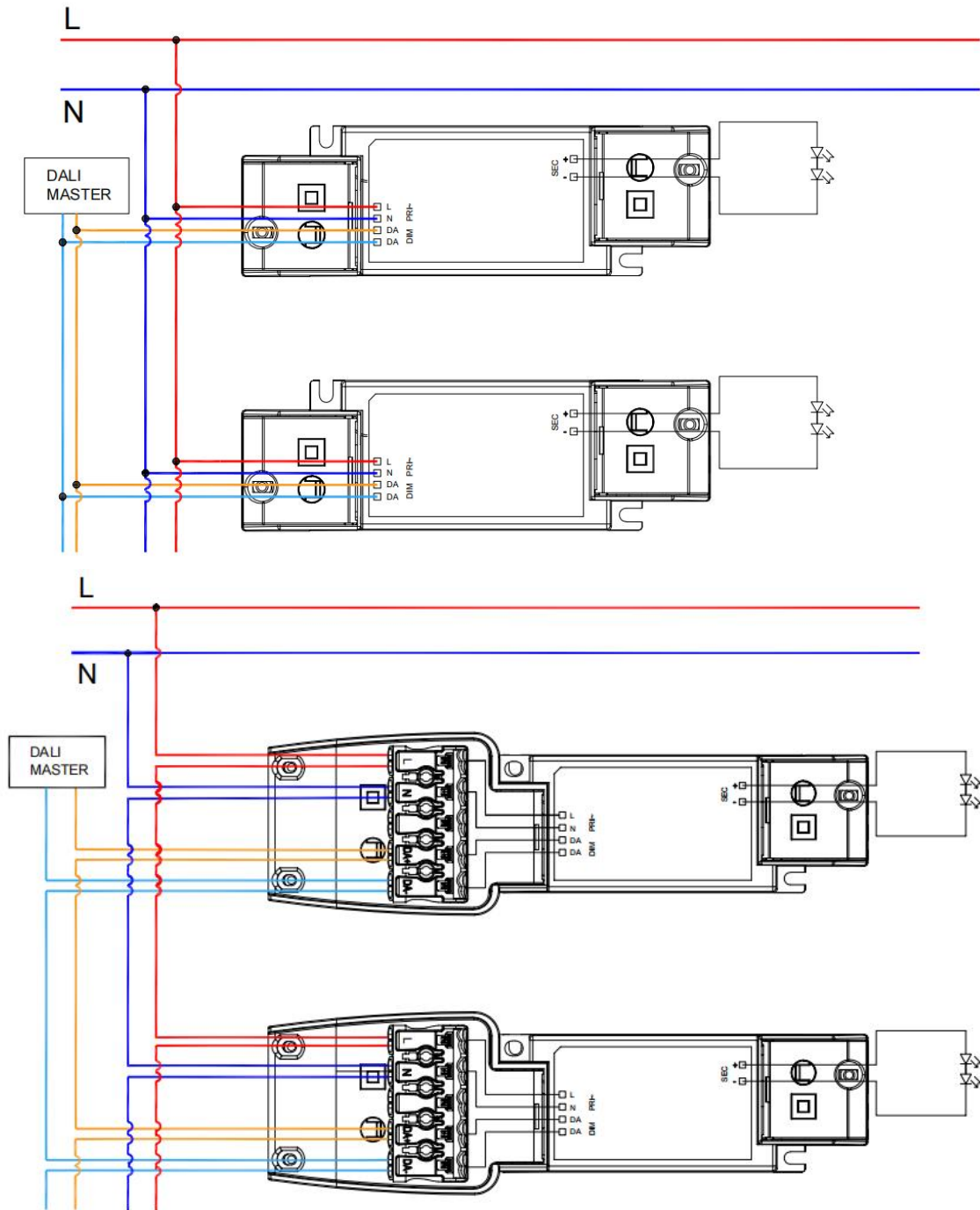
Fig. A: Dali Dimming
