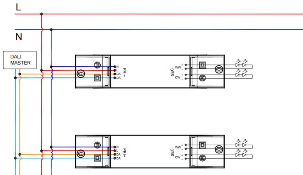
Fig. A: Push Dimming
