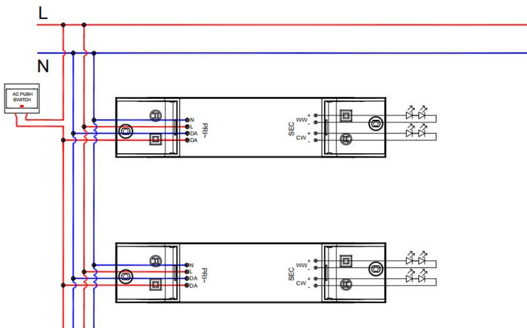
图A: Push 功能接线
